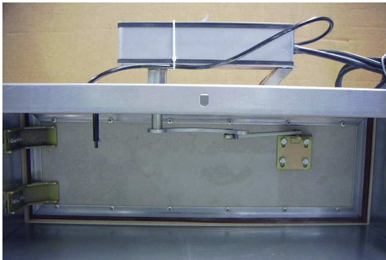
Ansicht Klappenflügel Kanalinnenseite - Antrieb
