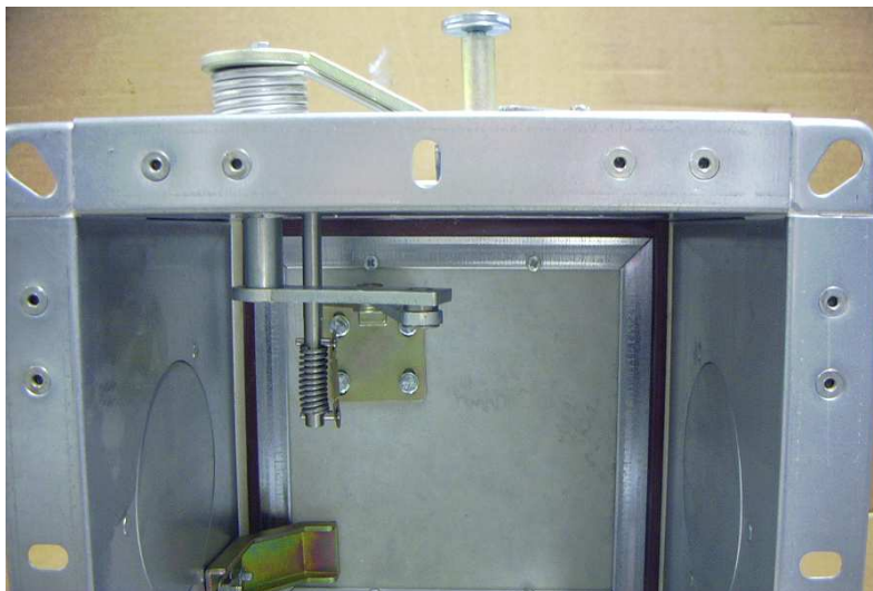
Ansicht Klappenflügel Kanalinnenseite Handauslösung
