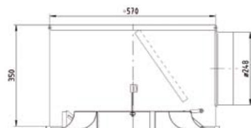
Coupe A-A avec plénum de raccordement
