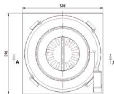
Diffuseur plafonnier IDA 600 sans plénum de raccordement
