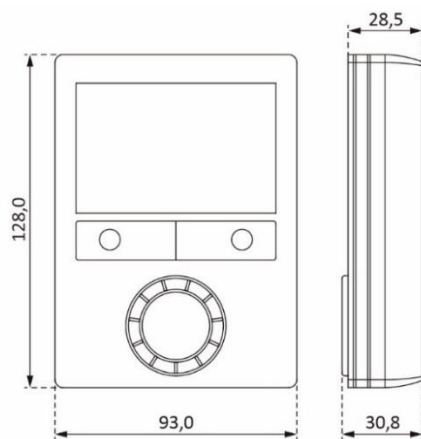
RDG...T-Modelle mit drei Auswahltasten
